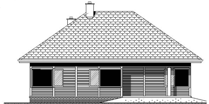
ELEWACJA OGRODOWA
